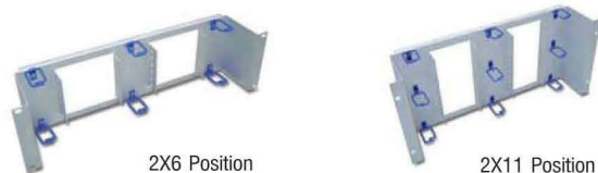
STG Rack Mount Back Mount Frame เป็นที่ติดตั้งได้กับตู้ Rack 19" มาตรฐานทั่วไป ใช้โมดูลที่ต้องการรวมบนโทรศัพท์เข้ากับระบบคอมพิวเตอร์ไว้ในตู้เดียวกันบนเครื่องข่ายคอมพิวเตอร์
