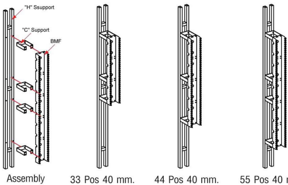
Back Mount Frame Set ประกอบด้วย Back Mount Frame ที่ประกอบเข้ากับ เสาเหล็กรูปตัว H พินสีน้ำตาลและแปะกึ่งตัวกันด้วย ใช้สำหรับติดตั้งในตู้ MDF ผนังที่พื้น
