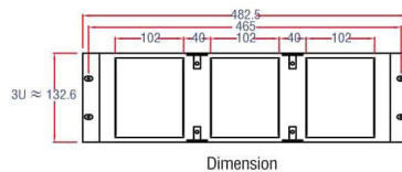
LSA+ Rack Mount Back Mount Frame ผนังที่ติดตั้งได้กับตู้ Rack 19" มาตรฐานทั่วไป ใช้ไม่กรณีที่ต้องพารวบรวมโทรศัพท์เข้ากับระบบคอมพิวเตอร์ไว้ในตู้เดียวกันกับเครื่องข่ายคอมพิวเตอร์
