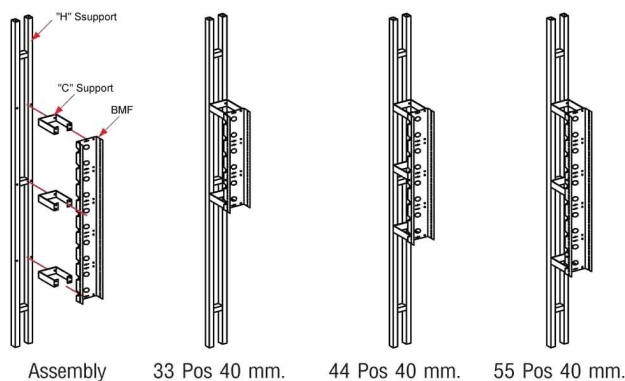
Back Mount Frame Set ประกอบด้วย Back Mount Frame ที่ประกอบเข้ากับ โครงเหล็กรูปตัว H พื้นสีเดียวกับโครงตู้โทรศัพท์ในตัวตู้ MDF มาตรฐานทั่วไป
